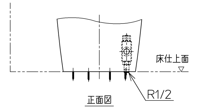
床給水仕様の場合
